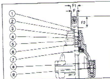
Zasuwa AVK – (7) – uszczelka zwrotna
