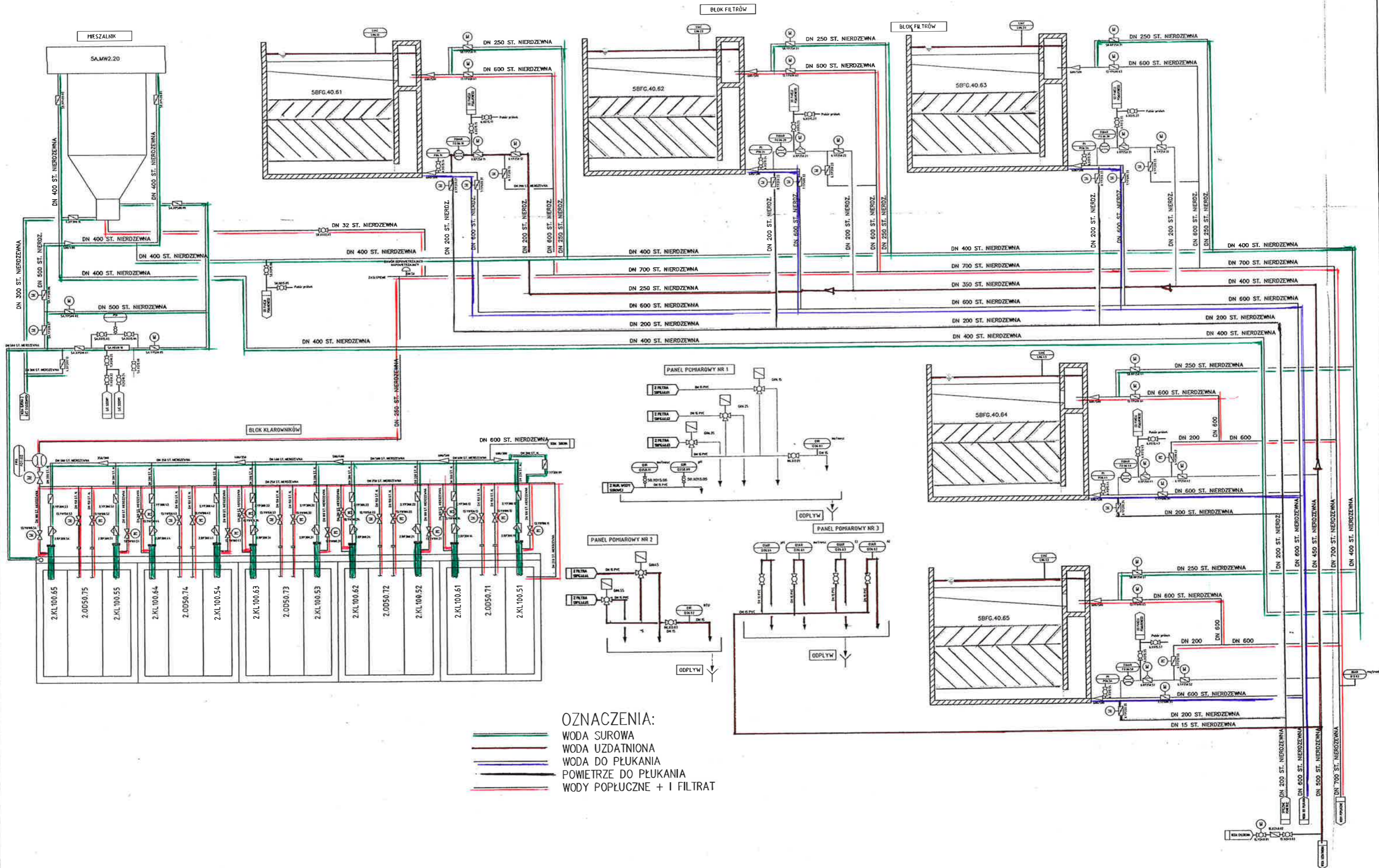
Rysunek nr 2. Schemat technologiczny filtrów i klarowników
